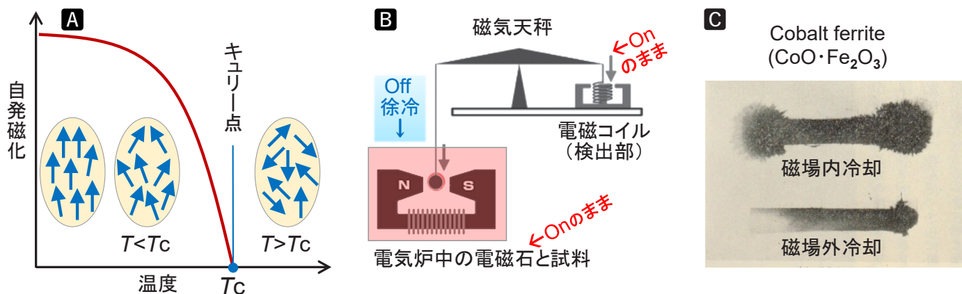
④ A , 磁性が消失する温度 T_c の決定と磁性体の磁区の向き。 B , 磁気天秤の原理と「磁場中冷却効果」の発見に至った時の装置の作動状況(青字と赤字)。 C , Hard ferrite(永久磁石)誕生の証拠写真。
