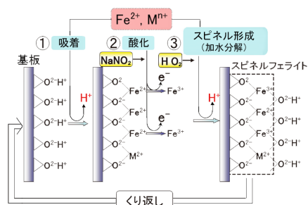
⑨ フェライトメッキの原理。 \text{Fe}^{2+} \rightarrow \text{Fe}^{3+} の酸化反応を利用して、フェライト薄膜を作製する〔出典：まてりあ 62, 588, 2023〕。
