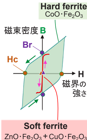
D: フェライトのB-H 曲線
