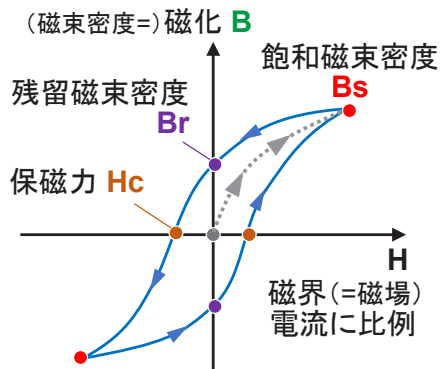
A: B-H 曲線(磁気ヒステリシス曲線)
